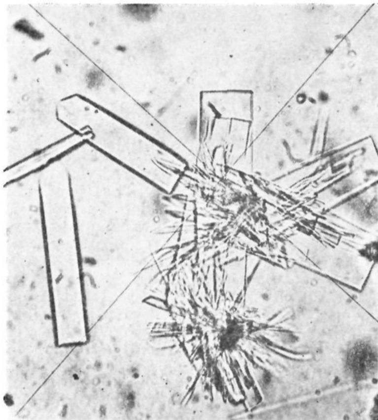
Fig. 1.— \beta -D-Isomaltose octaacetate.
